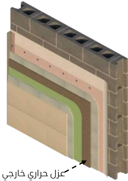
نظام حائط بالعزل الخارجي
