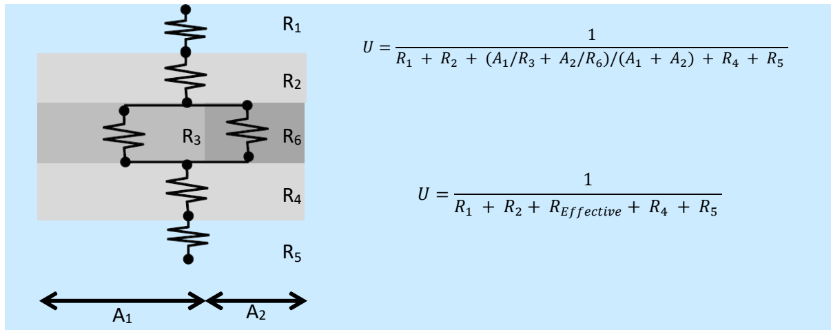
معادلة 5: معادلات حسب المسار المتحاور Isothermal Path Method
