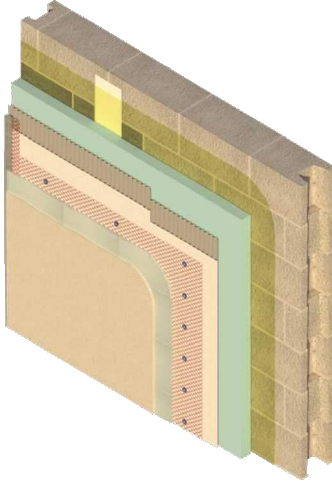
رسم توضيحي 12: مقطع هندسي لجدار مع طبقة مستمرة من العزل الخارجي
